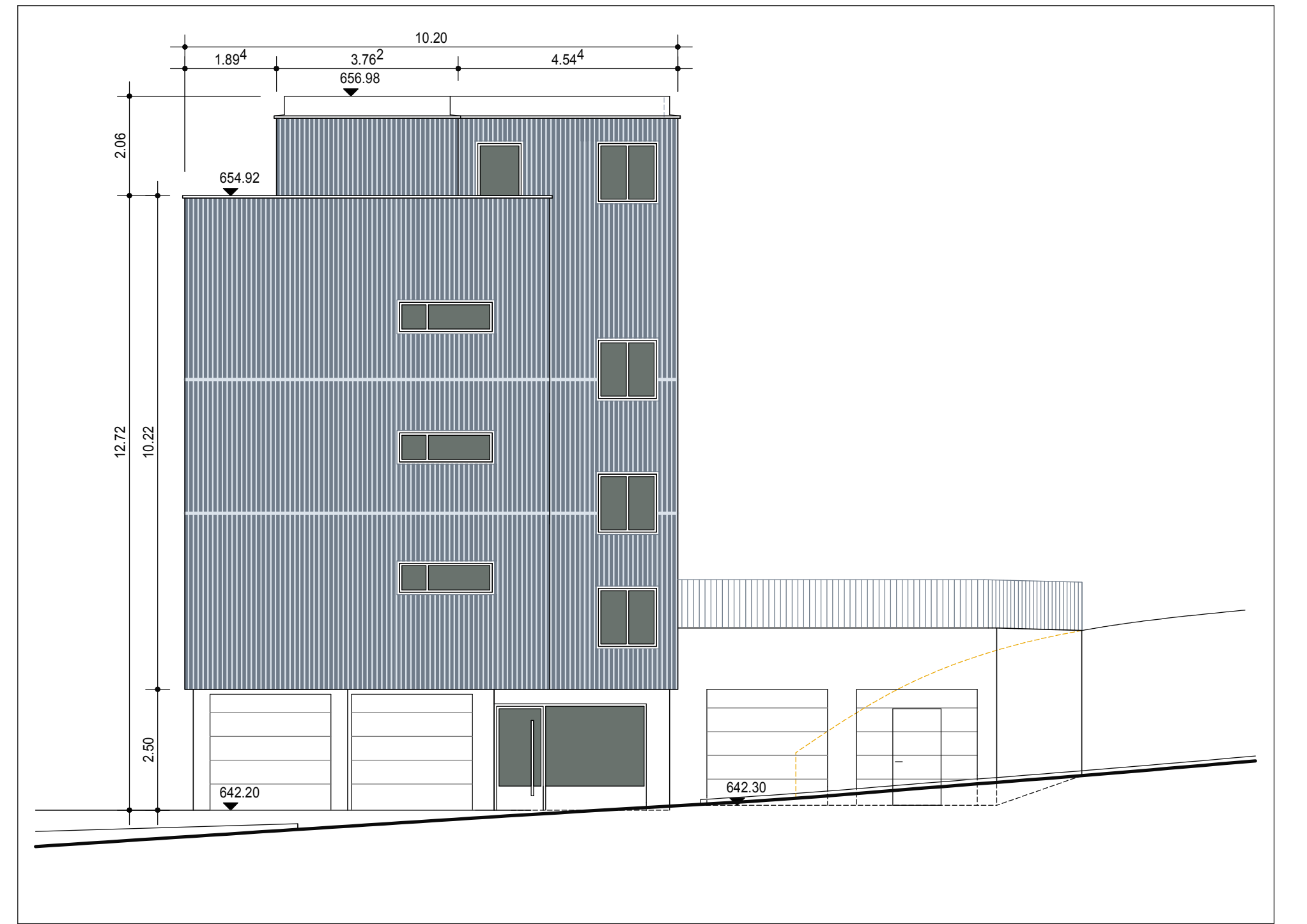
Ansicht Ost
