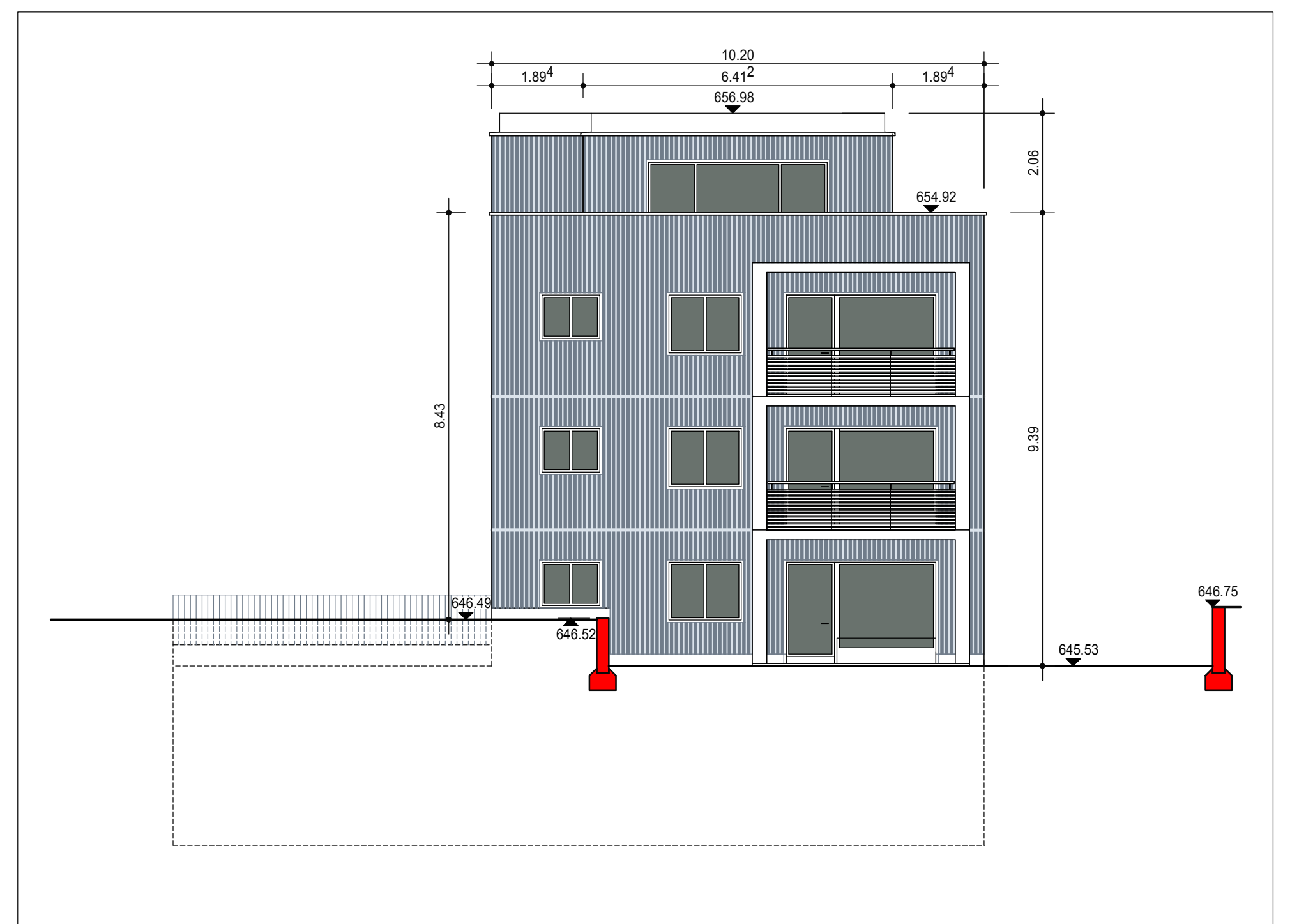
Ansicht West
