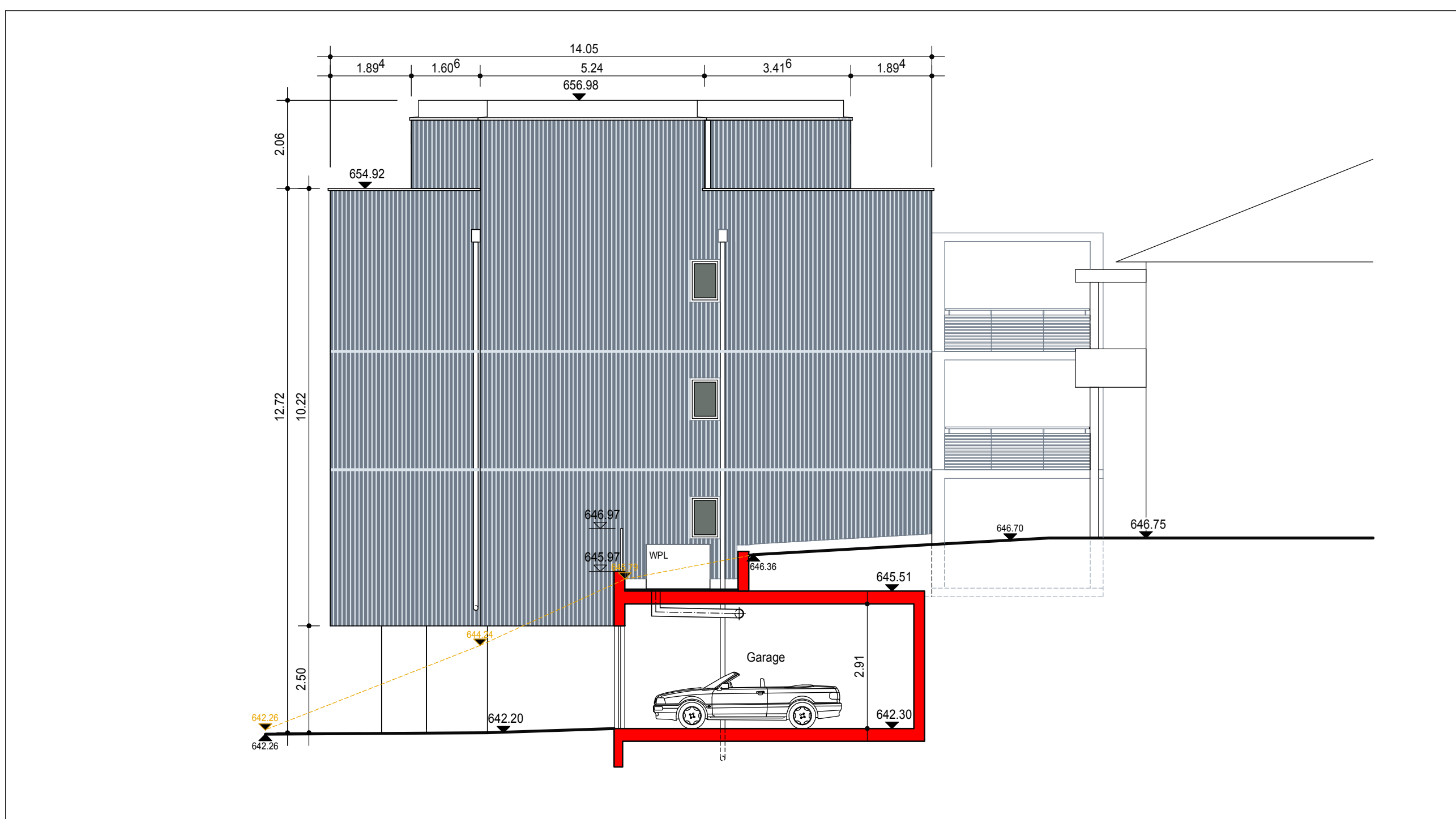
Ansicht Nord
